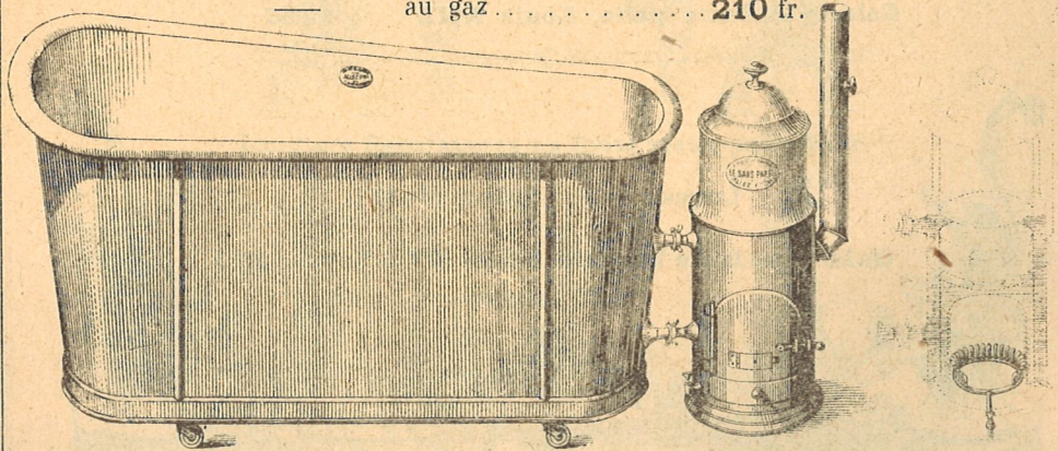
Baignoire marbrée à soupape et roulettes avec Chauffe-Bain le "SANS-PAREIL" , Breveté S. G. D. G. Propriété exclusive de la maison.
